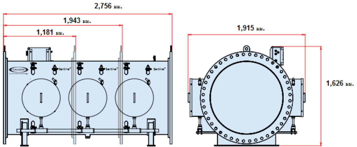
มิติขนาดของเครื่องรุ่น SENTINEL® 48
