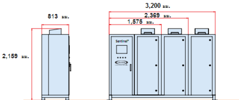
มิติขนาดของตู้ควบคุม SENTINEL® 48
